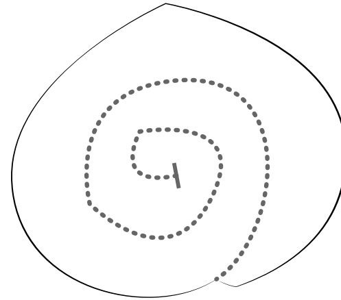
Spiralantenne
